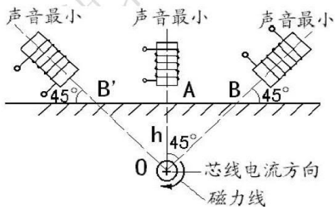
80%法测深示意图
