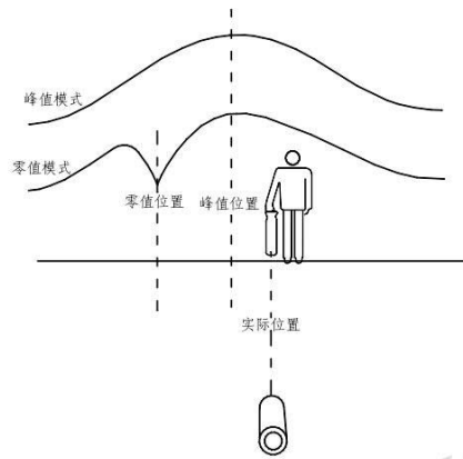
零值法和峰值法探测比较示意图
