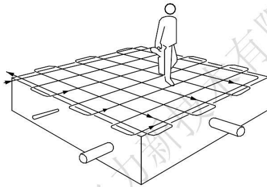
被动源工频法示意图
